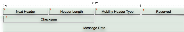
Fig. 9. Format du Mobility Header (MH)
