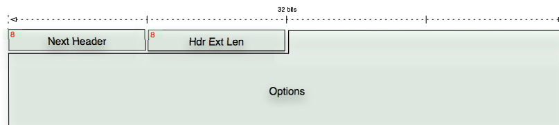
Fig. 3. Header IPv6
