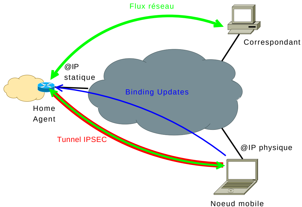
FIG. 6: Fonctionnement de Mobile IPv6.
