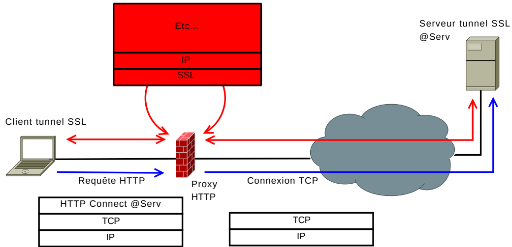
FIG. 1: Exemple de lien VPN SSL utilisant la méthode CONNECT.
