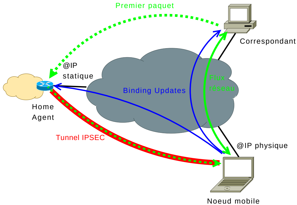
FIG. 7: Fonctionnement optimisé de Mobile IPv6.
